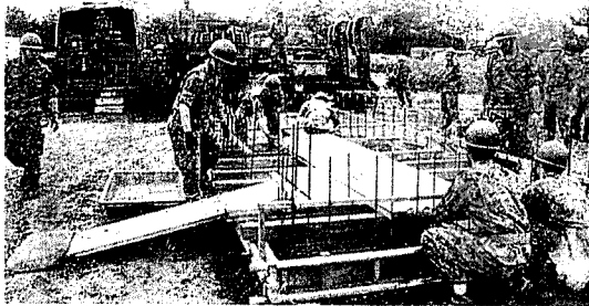
コンクリート構築訓練
